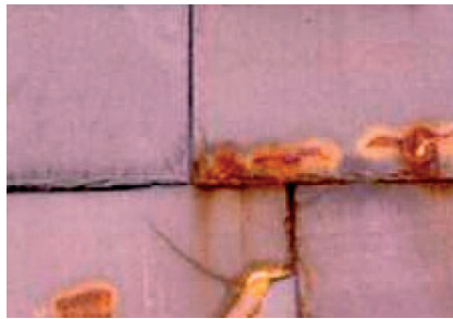
Figur 2. Nedbrydning af skifer med for stort jernindhold. Skaden kunne være undgået, hvis stenene havde været kvalitetsprøvet med fortyndet saltsyre inden oplægning.
