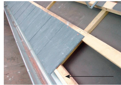
Figur 3. Pilen viser "skiferlisten", som monteres ved tagfod (og tagrygning) for at undgå at skiferstenene vipper.
